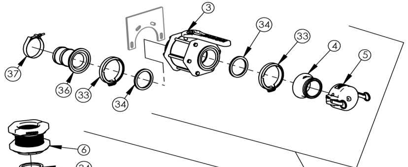
3" BOTTOM FILL
