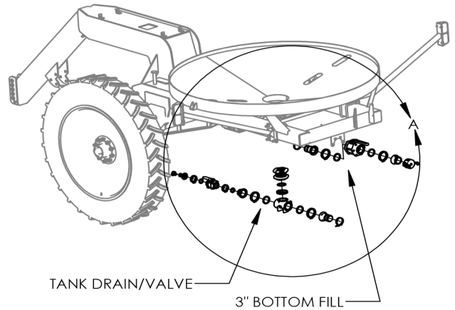
3" BOTTOM FILL
